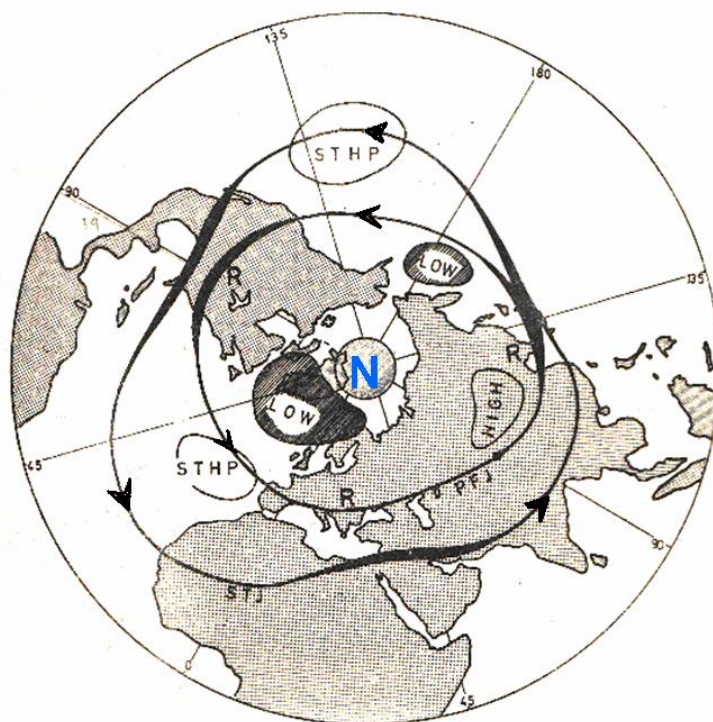
شکل ۸. گردش بادهای سیاره‌ای (رودباده‌ها) حول قطب شمال با اثر نیروهای منحرف کننده [۱۲].
